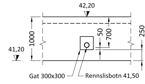
Skýringarmynd af sökkulgötum
